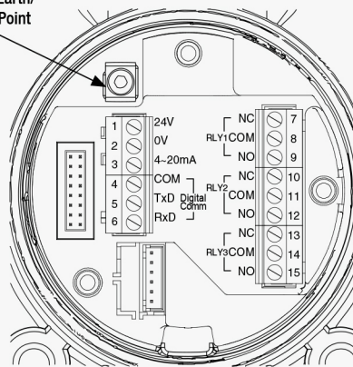
Terminal Module
